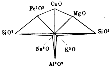
Fig. 6. Melaphyr von Palle rabbiose (DOELTER analys.) 1 .
